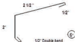
DRIP EDGE FLASHING - 6"
